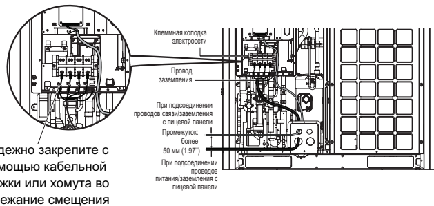
Подсоединение провода связи/заземления
