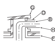
Ввод в зоне с повышенными противопожарными требованиями и ограждающей стеной
