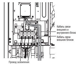
Подсоединение провода связи/заземления
