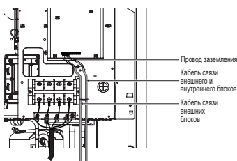
Подсоединение провода связи/заземления
